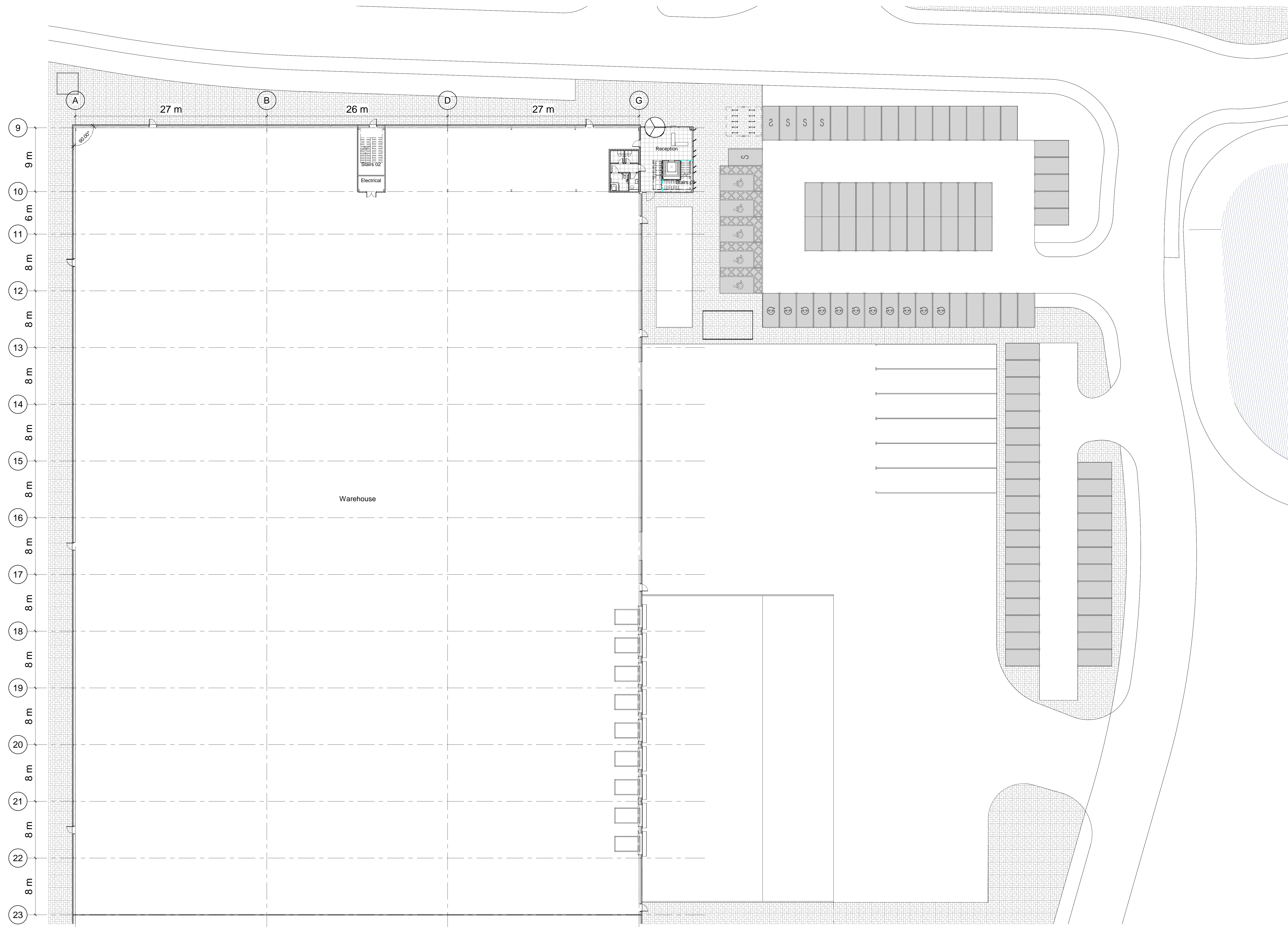
1 Site Layout 1 : 200
